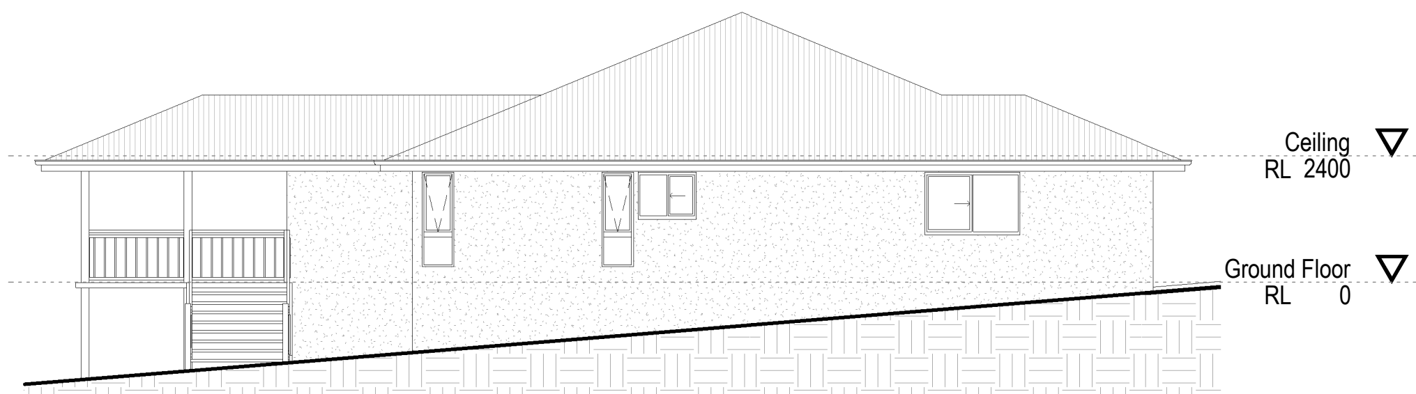
4 SW Elevation 1 : 100
