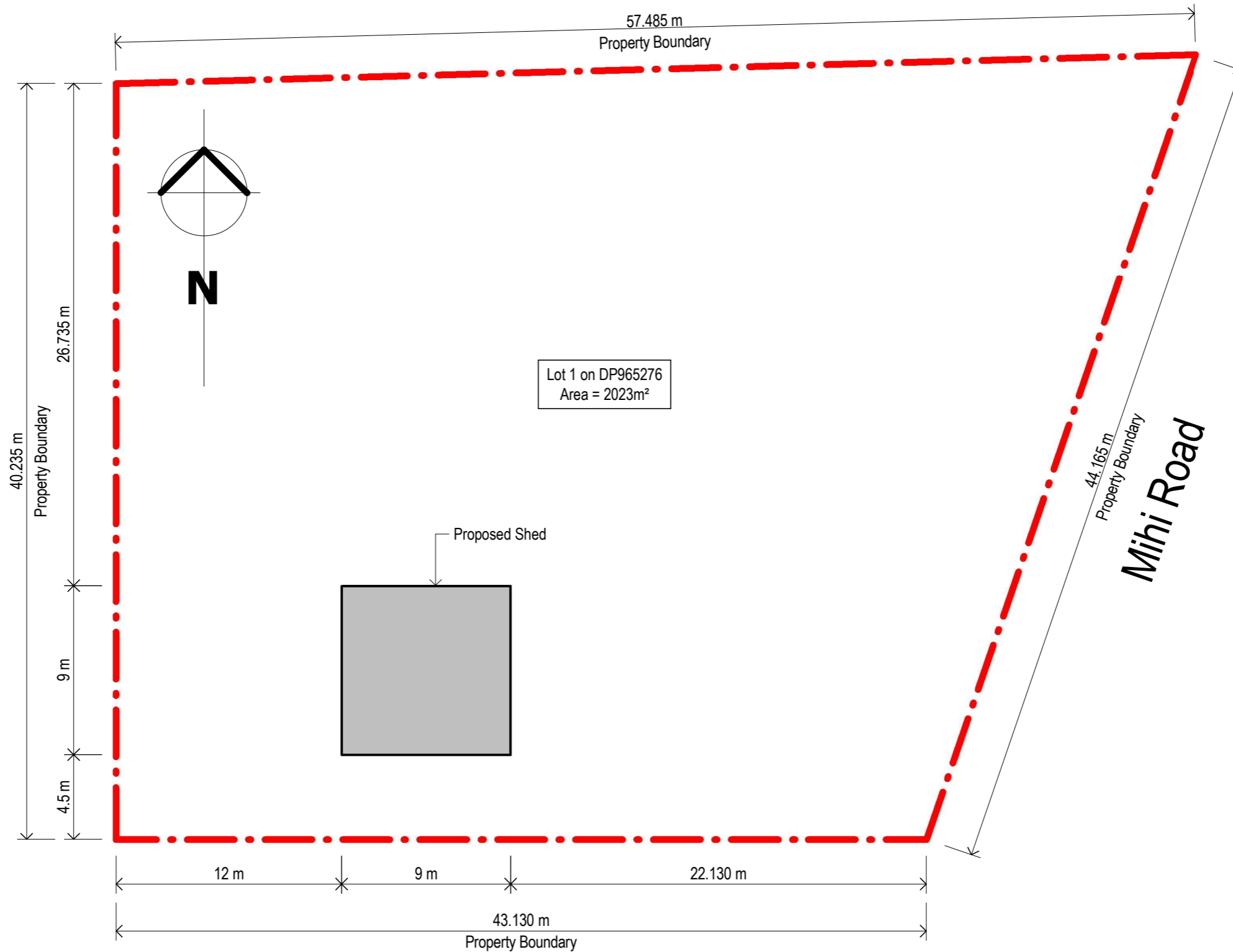
1 Site Plan 1 : 250
