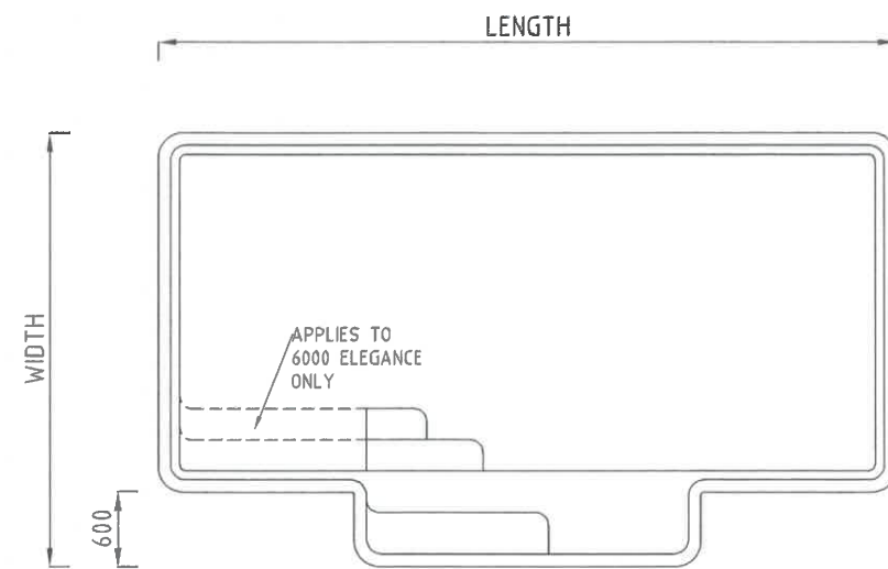
POOL PLAN - ELEGANCE N.T.S
