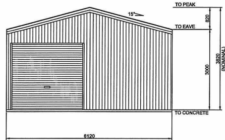
4 6 ENDWALL EXTERIOR ELEVATION SCALE: 1 = 100
