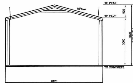
3 6 ENDWALL EXTERIOR ELEVATION SCALE: 1 = 100
